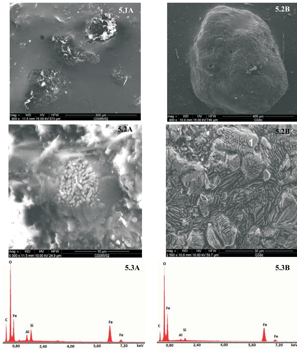
Rys. 5. Analizy SEM/EDS niejednorodności na powierzchni badanych pastylek
