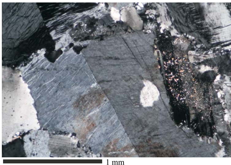
Rys. 1. Mikroperyt mikroklinowy z plamiście rozłożonym pigmentem, zserycytowany plagioklaz, kwarc. PX
