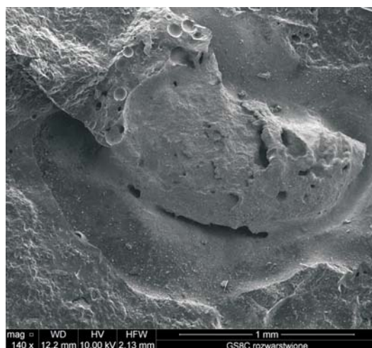
Rys. 9. Rozwarstwienie powstałe w pastylce nr 2 w trakcie szlifowania. SEM
